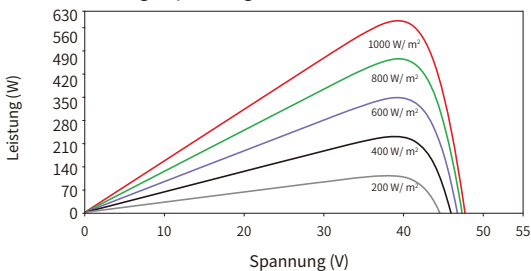
Leistungs-Spannungs-Kurven (66HL4M-(V) 615W)
