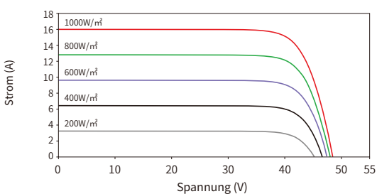
Strom-Spannungs-Kurven (66HL4M-(V) 615W)
