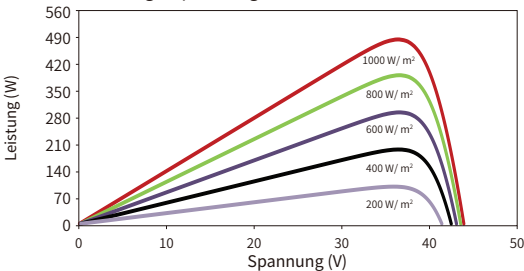
Leistungs-Spannungs-Kurven (60HL4-(V) 490W)
