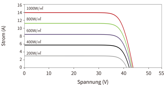
Strom-Spannungs-Kurven (60HL4-(V) 490W)
