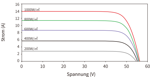
Strom-Spannungs-Kurven (78HL4-BDV 640W)
